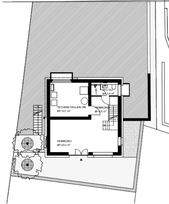
UNTERGESCHOSS
